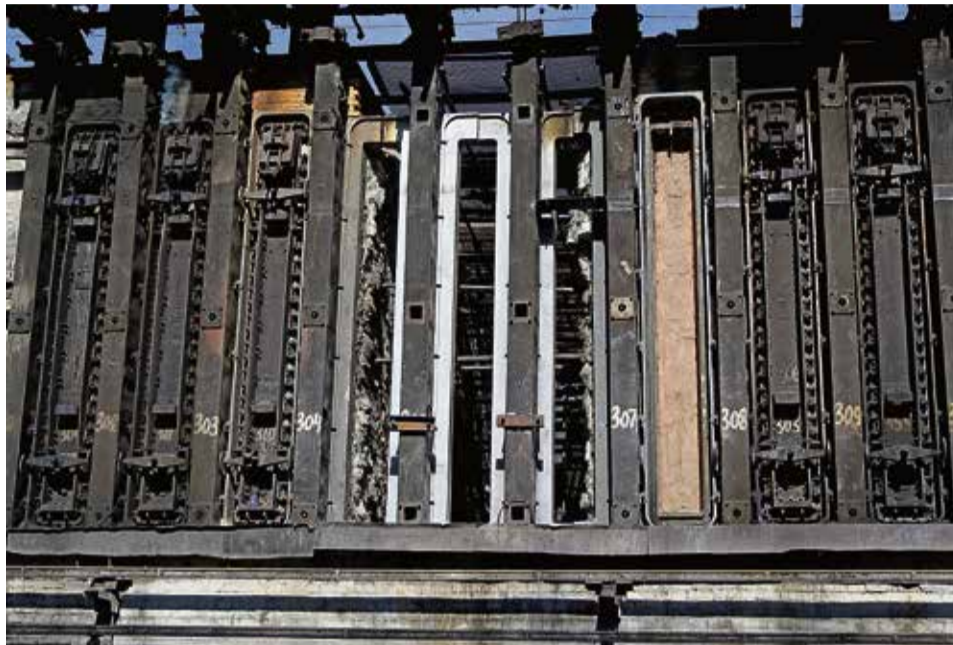
▲ Ремонт отдельной ячейки коксовой батареи не приводит к остановке всего комплекса, а значит, доменщики не испытывают дефицита в топливе для своих печей
